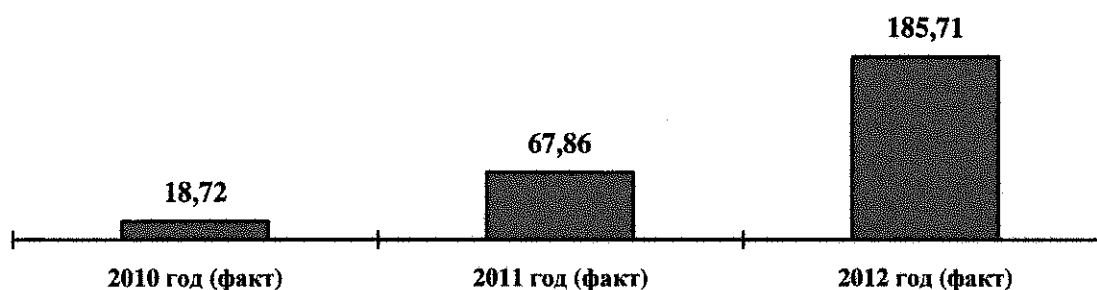
Рис. 41. Поступление платы за пользование водными объектами в федеральный бюджет, млн. руб.
